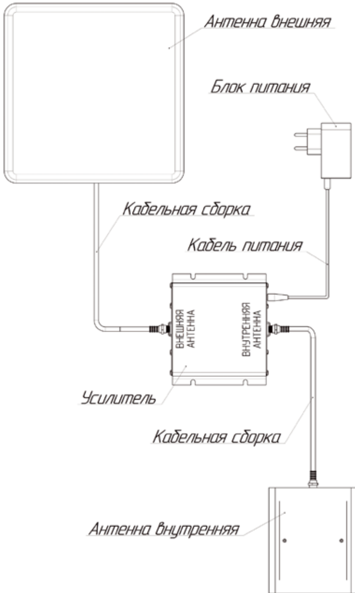
Рисунок 6. Схема подключения
